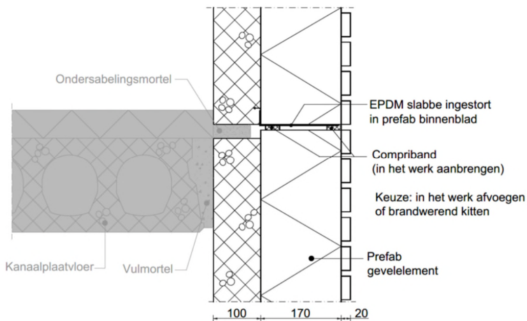
Figuur 6 – Detail verdiepingsvloer langszijde met kanaalplaatvloer
