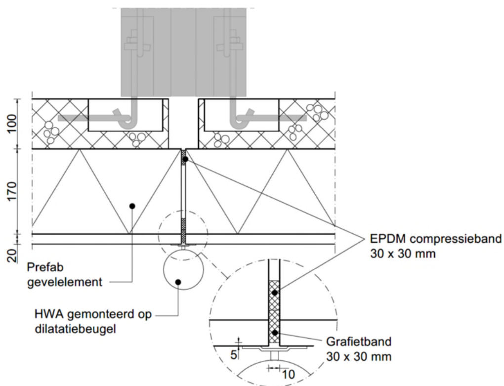
Figuur 9 – Verticale naden tussen twee gevelelementen voorzien van geprefabriceerde compressiebanden
